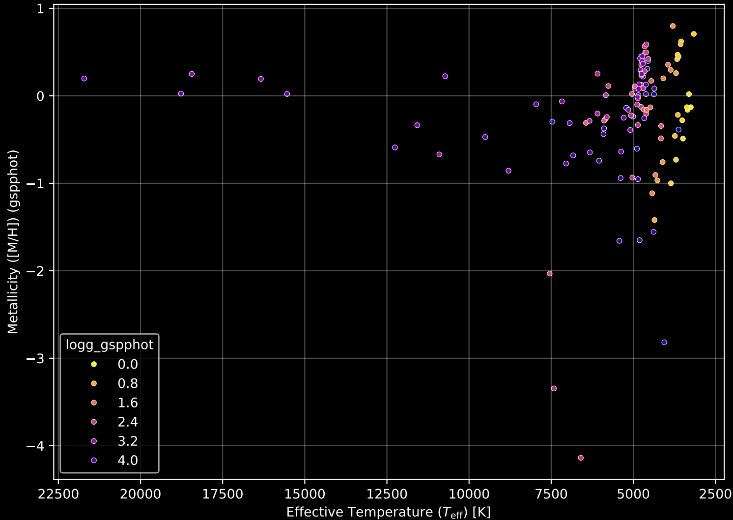
APOGEE DR17 Field: [022+00] Stellar Population Parameters (n= 122)
